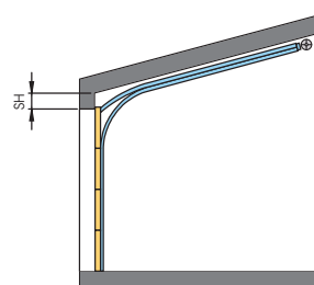
Niedrigsturzsystem mit Dachfolge
