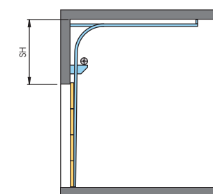
Höherführung mit Vierkantrohr SH min. 2000
