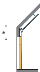
Standardsystem mit Dachfolge bis 45°
